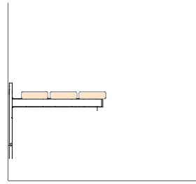
dress-6210 - Bankkonsole mit Wandbefestigung wall-mounted bench panel
