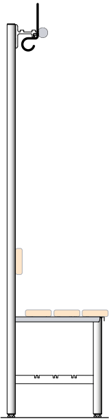
dress-6x70 - einseitige Umkleidebank mit Garderobe, mit Rückenlehne, Schuhrost optional. Haken frei wählbar dress-6670 - one-sided changing room bench with coat rack, backrest, optional shoe rack. Free choice of hooks
